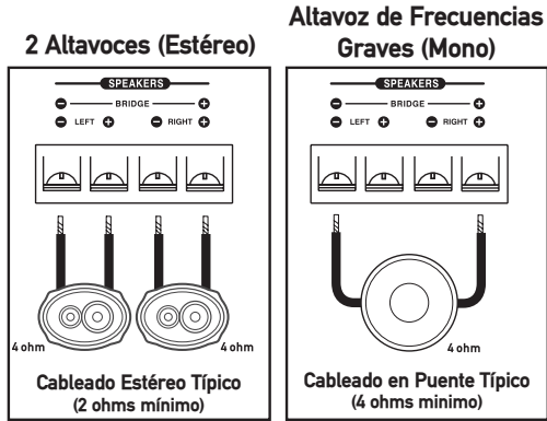
XPA2500 conexiones del altavoz
