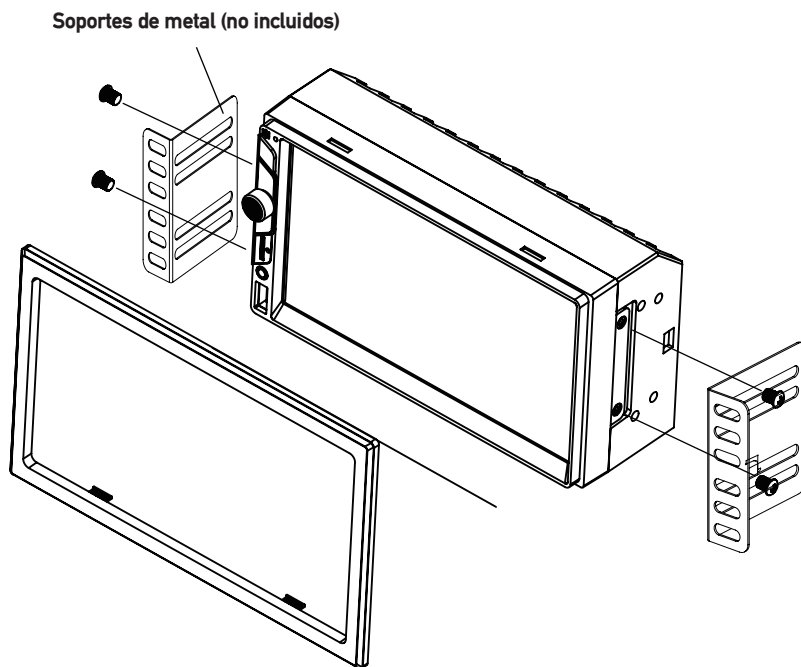
METODO DE MONTAJE TIPICA DE CARGA FRONTAL
