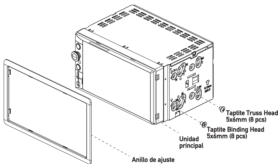
Método de montaje típica de DIN y carga frontal
