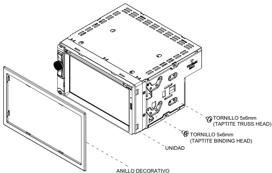
METODO DE MONTAJE TIPICA DE CARGA FRONTAL
