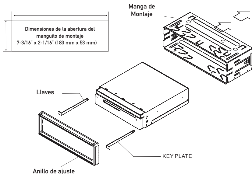
MÉTODO DE MONTAJE TÍPICA DE CARGA FRONTAL
